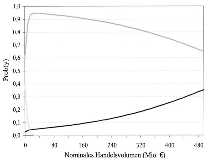
Abbildung 6: Wahrscheinlichkeit der Ausführung einer Transaktion über die Präsenzborse (hellgraue Linie), OTC-bilateral (dunkelgraue Linie) und OTC-maklervermittelt (schwarze Linie) in Abhängigkeit des nominalen Handelsvolumens
