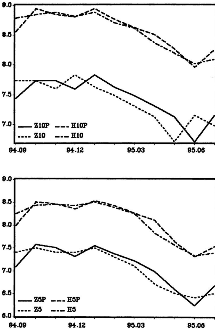
Abb. 7: Ein-Schrittprognosen auf Grundlage des kompletten Systems
