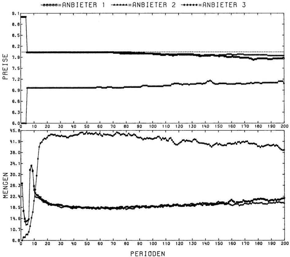
Abb. 4: Homogene Marktbeseztung Modell C, verschiedene Anfangsbedingungen
